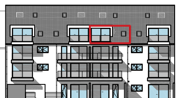
Parkview 1 - Ommegangstraat / ACHTERGEVEL
